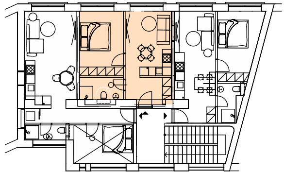
SITUÁCIA 2.NP - APARTMÁNU Č.C.2
