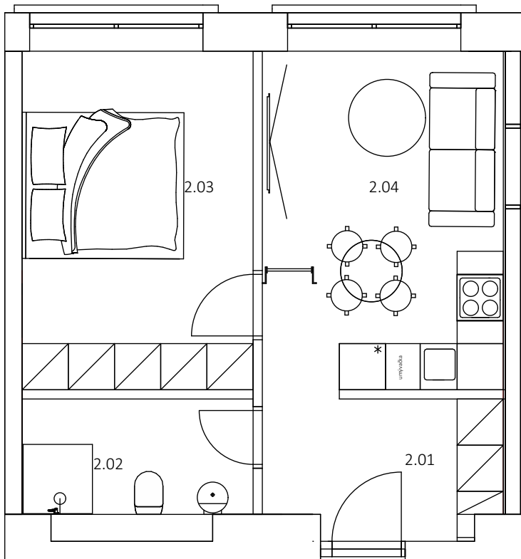
PÔDORYS APARTMÁNU Č.C.2
