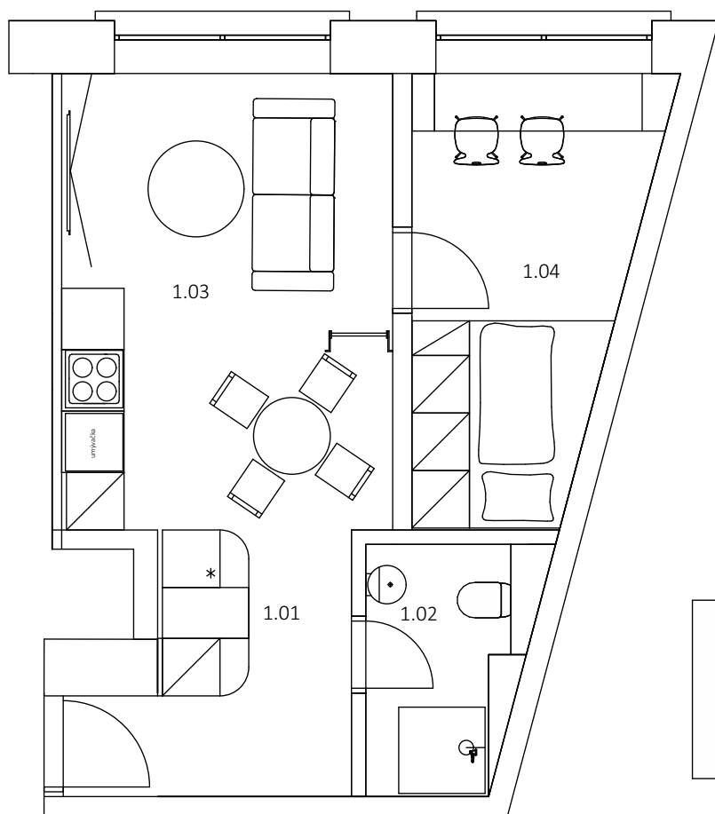
PÔDORYS LOFTOVEJ ČASTI
